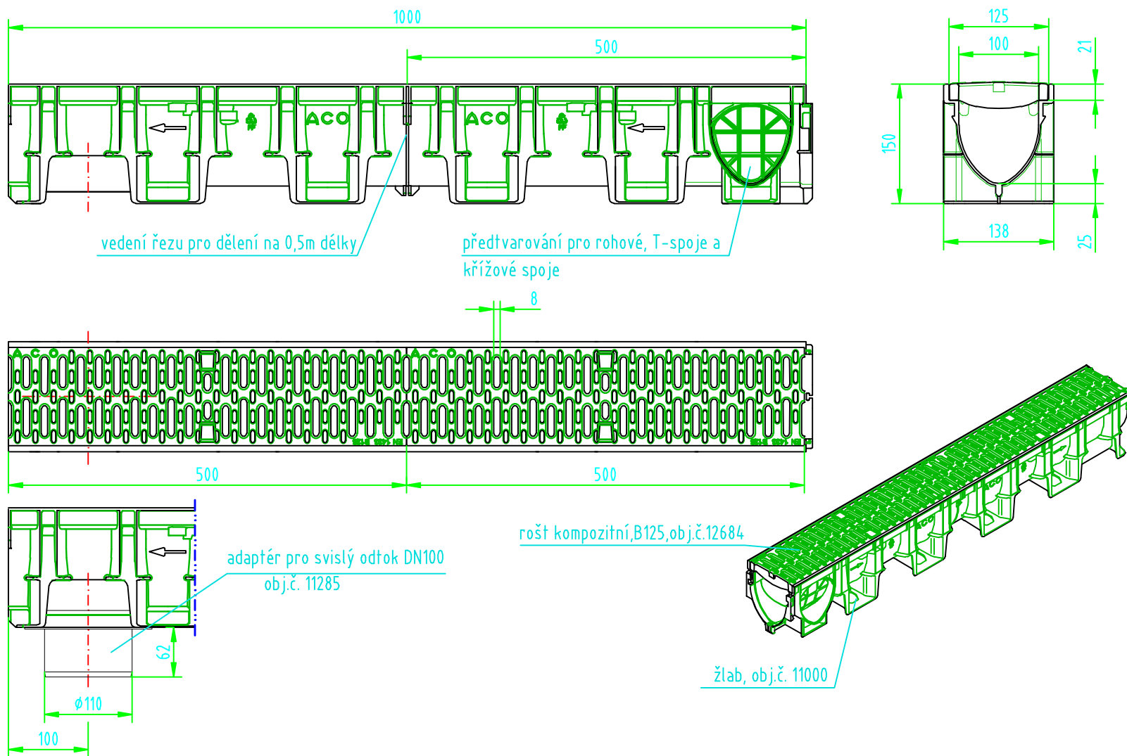
ACO DRAIN X 100 C - žlab H=150mm s kompozitním roštem B125kN
